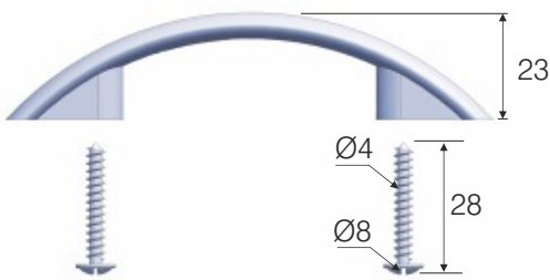
Plastik için özel dişli vida Special threaded screw for plastic специальный винт для пластика
